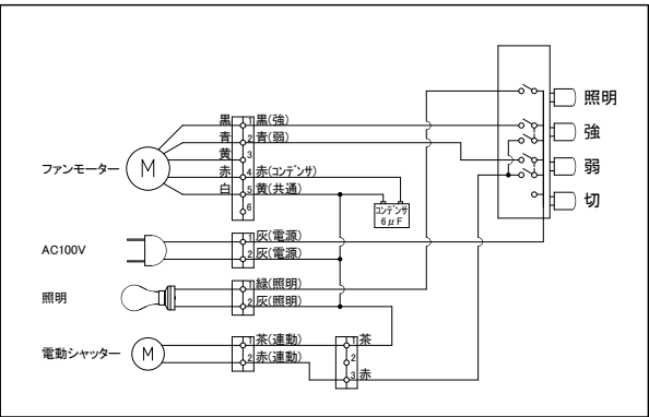
□結線図
