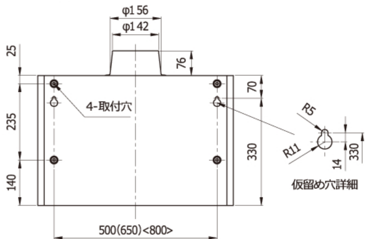
背面取付図
