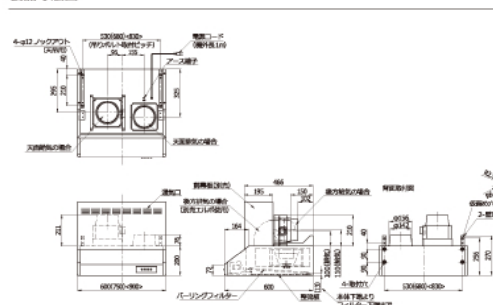
製品寸法図
