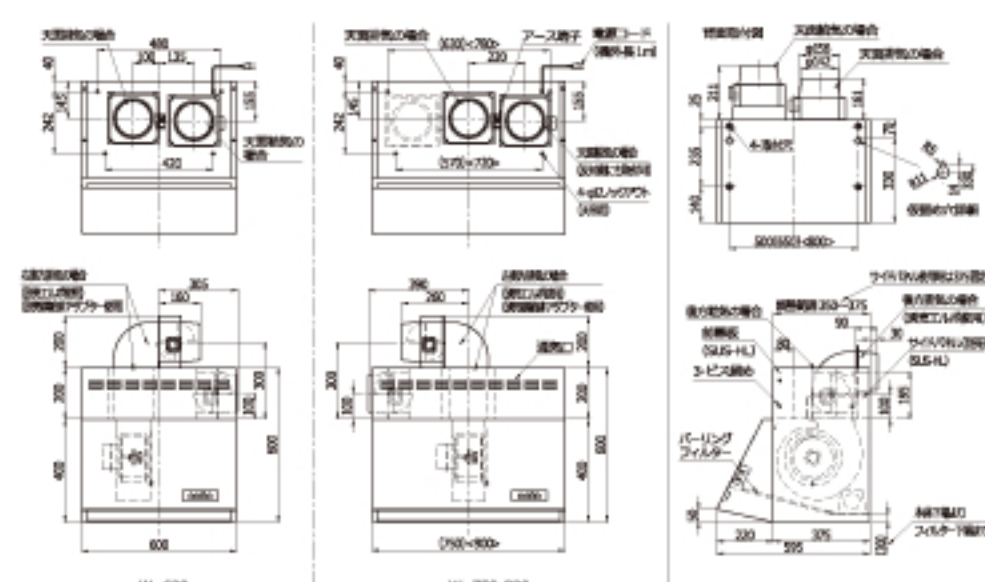
製品寸法図
