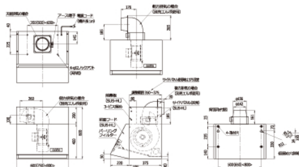
製品寸法図
