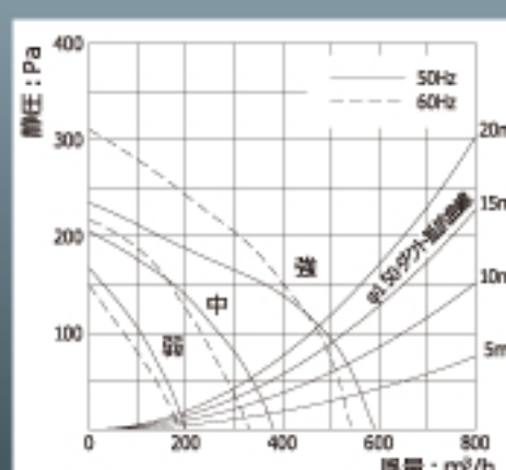
静圧・風量曲線
